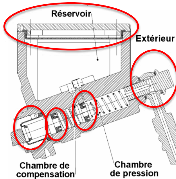
Éclaté du Maître-Cylindre de frein avant (à compléter)
