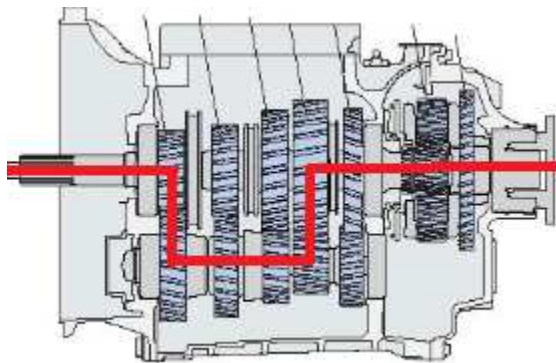
Chaine cinématique en 7 ème
