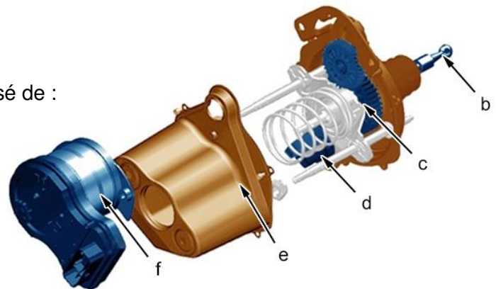
(1) Amplificateur de freinage électrique. "a" Connecteur 26 voies noir.
