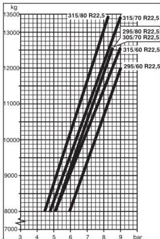
Montage jumelé
