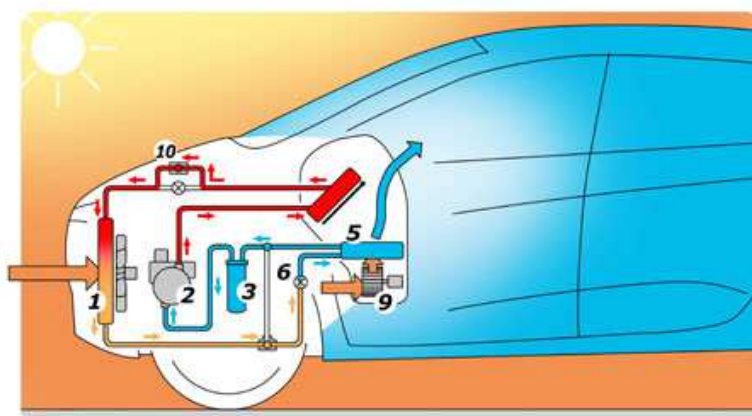
Circuit en mode climatisation
