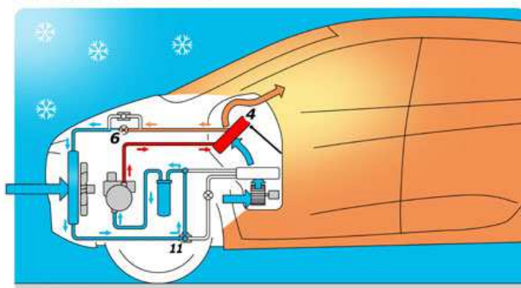
Circuit en mode chauffage
